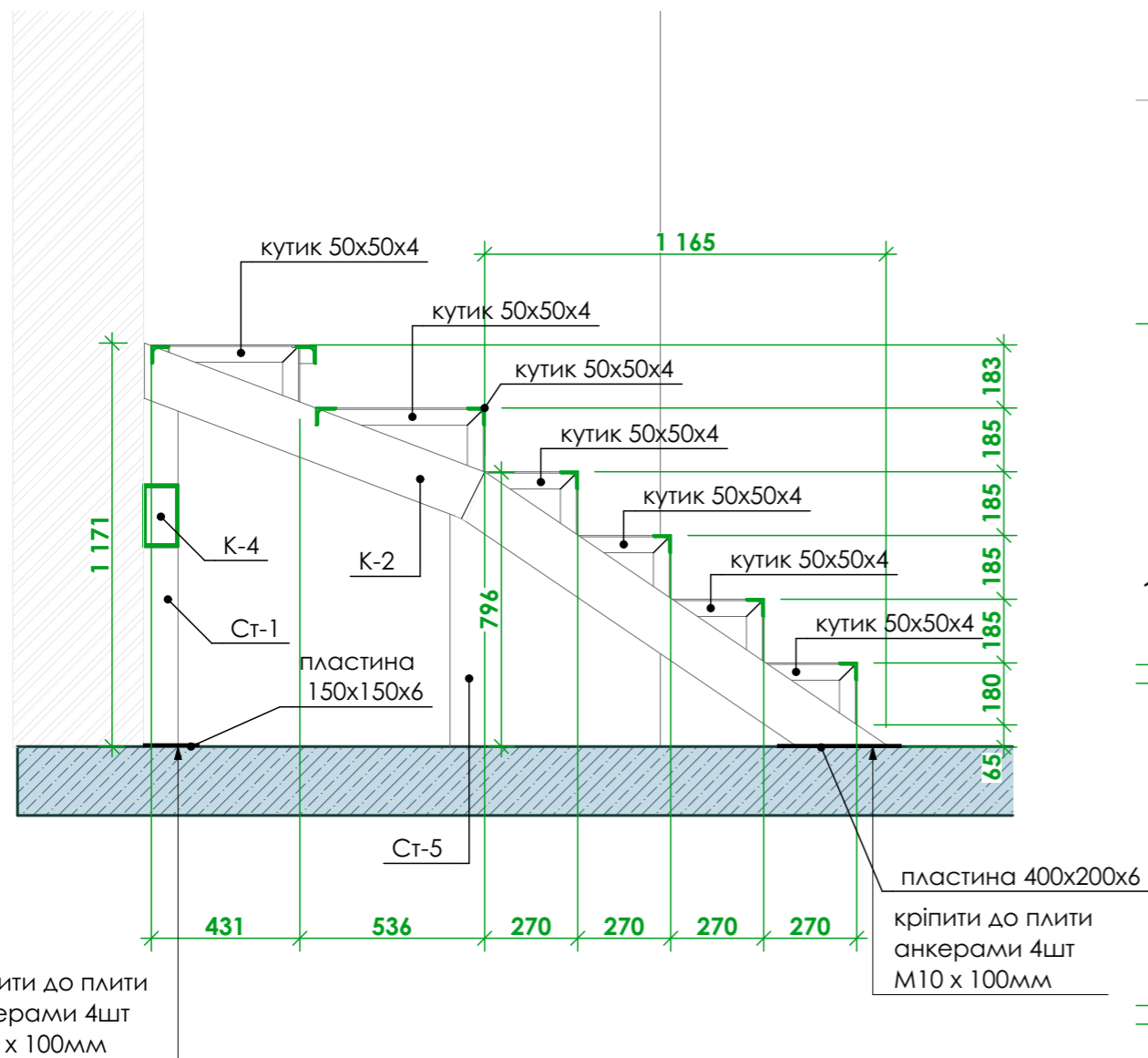
Схема розміщення косоурів
